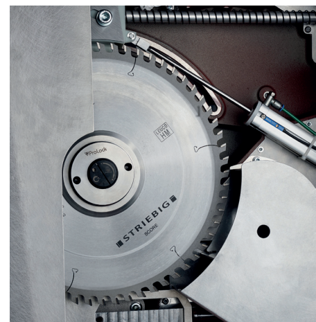
Verbesserte Standard-Ausstattung für Standard S, Edition 60, Evolution und Control: das Prolock Easy-Fix Werkzeugspannsystem bietet eine einfache, robuste und präzise Handhabung.
