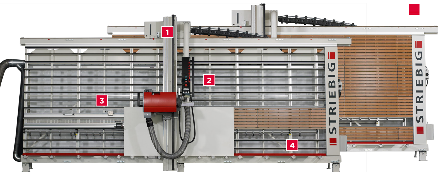
Abb.: STRIEBIG STANDARD S - in zwei Ausführungen: TRK2 mit Alulattenrost, TRK1 mit Holzauflegewand
